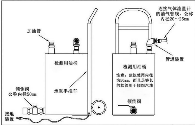
图C.2 检测用油桶部件安装示意图
