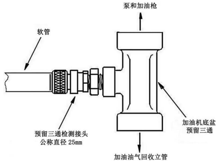
图 A. 2 三通检测接头示意图
