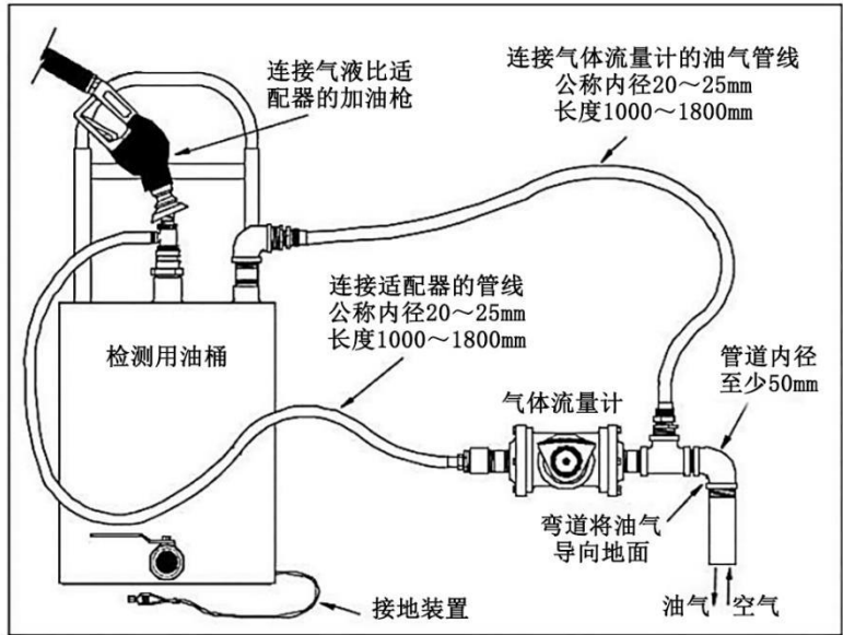
图C.3 气液比检测装置安装示意图
