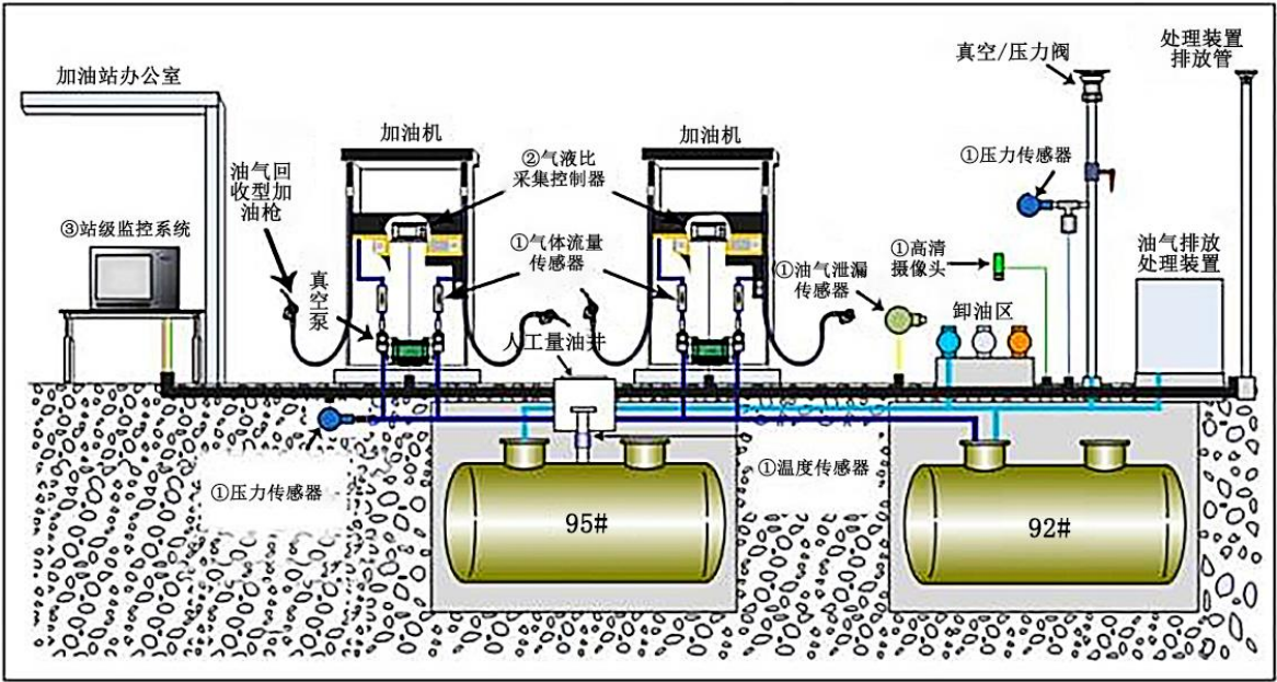
图 E.1 在线监测系统
