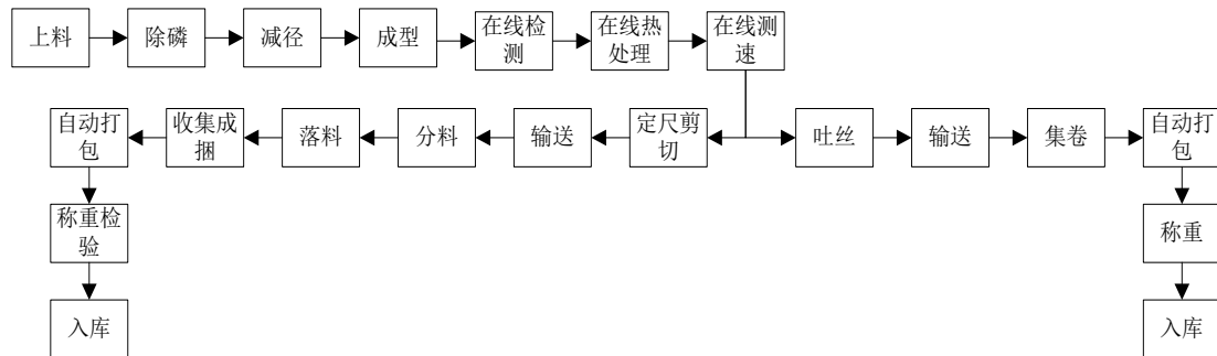
图 8-1 高延性新型冷轧带肋钢筋工艺流程
