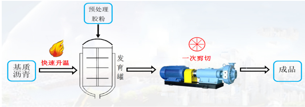
图 7-1 工艺流程图
