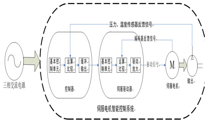
图 5-1 系统控制原理图
