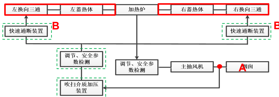
图 4-1 工艺流程图
