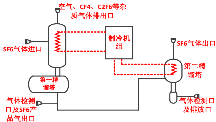
图 11-3 双塔精馏提纯工艺流程图
