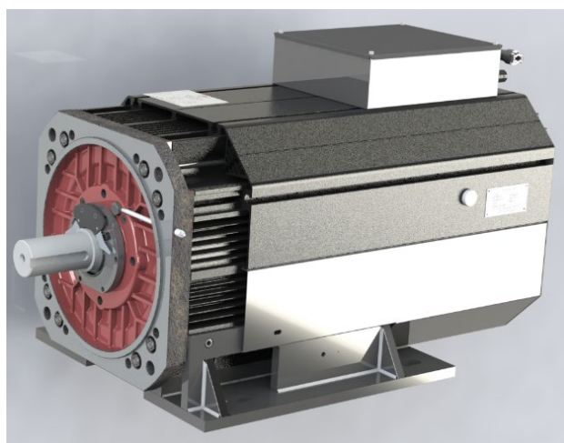
图 5-3 电机外观
