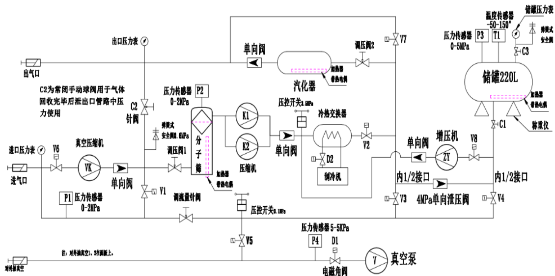
图 11-2 六氟化硫净化处理工艺流程图
