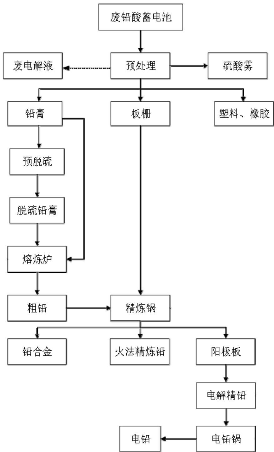
图 13-3 再生铅典型生产工艺流程图
